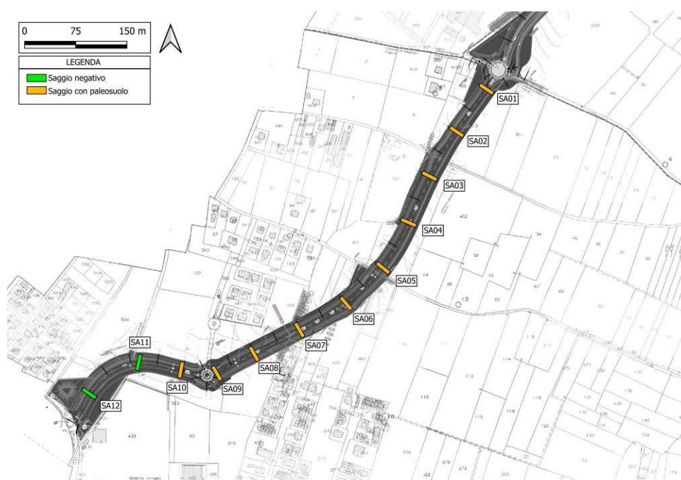
Figura 4 – Planimetria di progetto su catastale con posizionamento dei saggi archeologici
